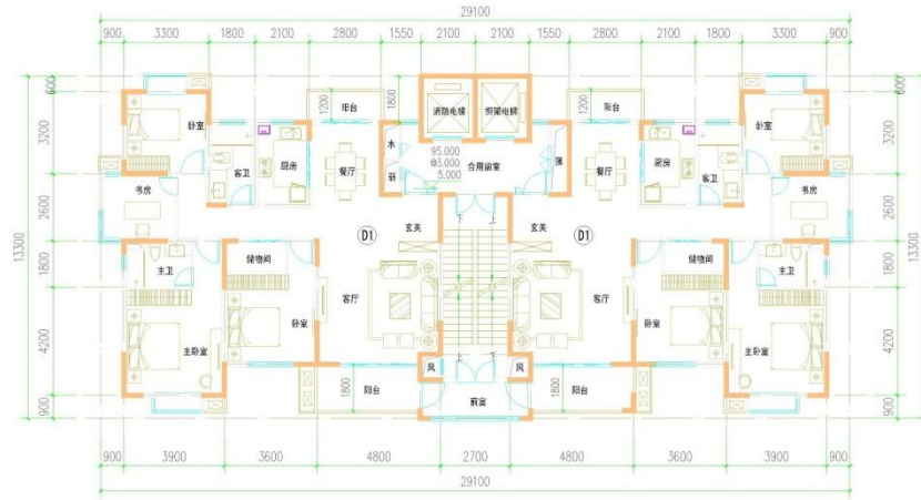
13#、15#、18#楼标准层平面图
